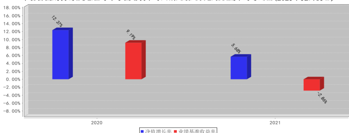
平安价值成长混合C基金每年净值增长率与同期业绩比较基准收益率的对比图(2021年12月31日)
